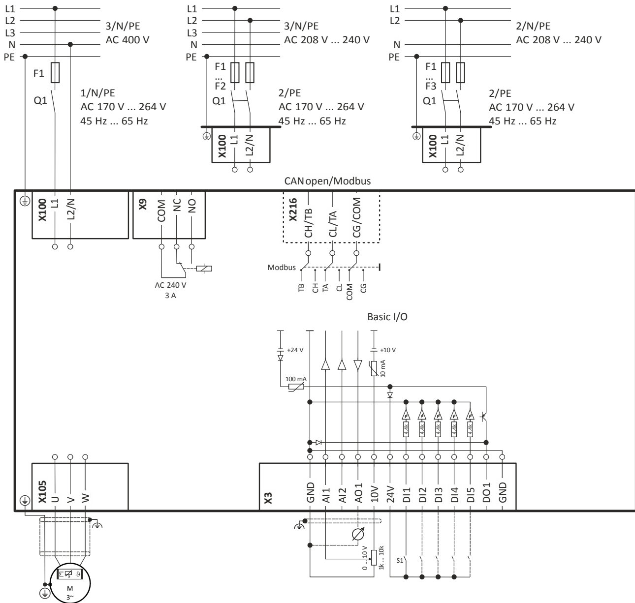
Fig. 2: Wiring example
