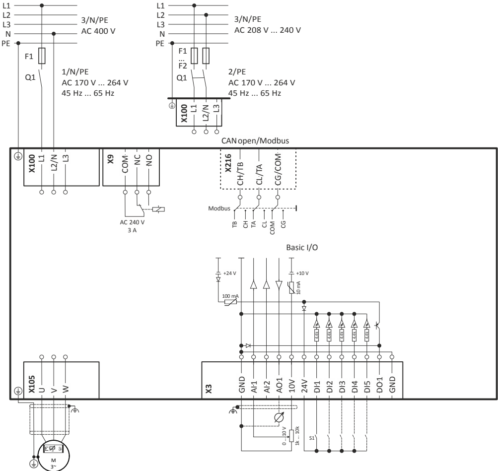
Abb. 2: Anschlussbeispiel
