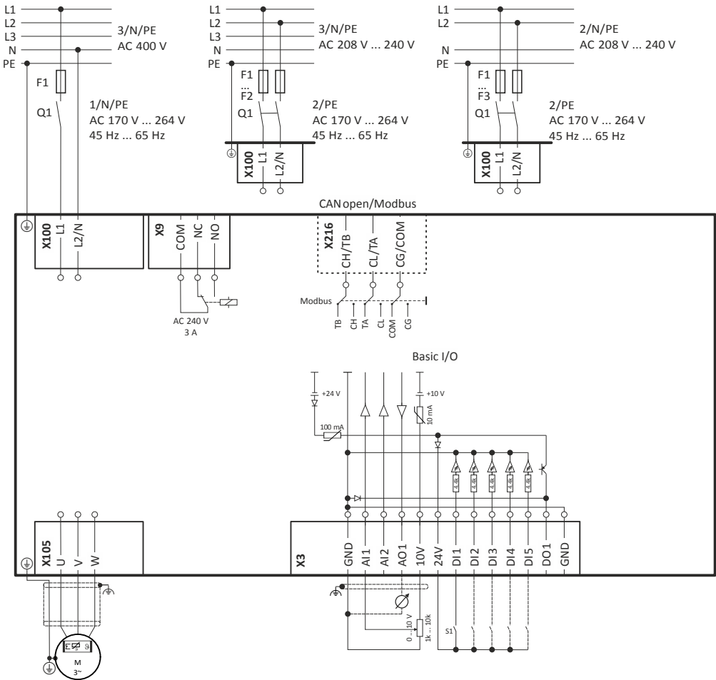
Abb. 1: Anschlussbeispiel
