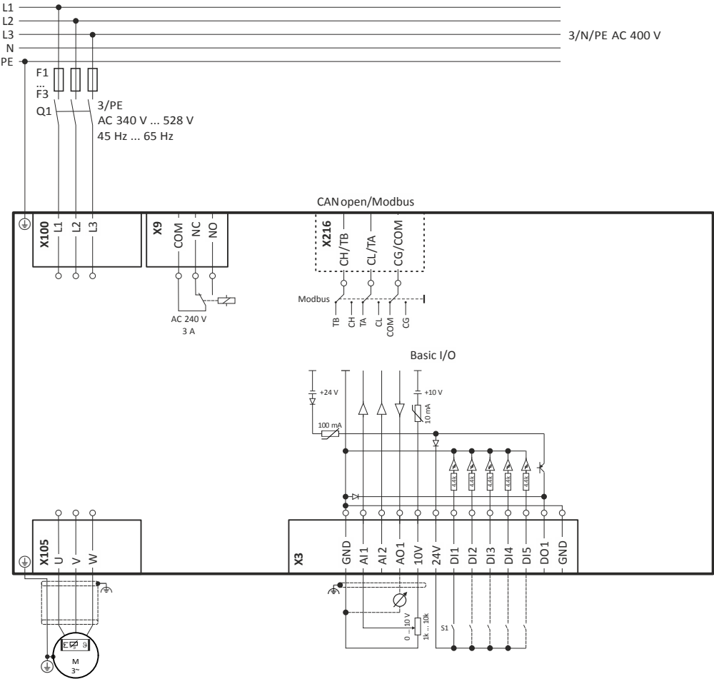
Abb. 5: Anschlussbeispiel
