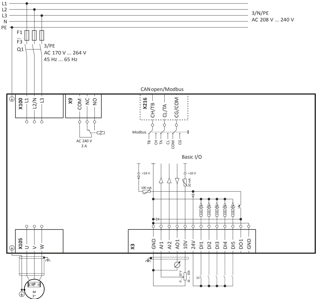
Abb. 4: Anschlussbeispiel
